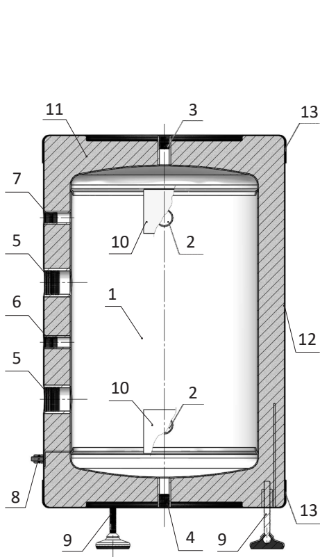
Obr. 1 AKU ST 50 S - popis
