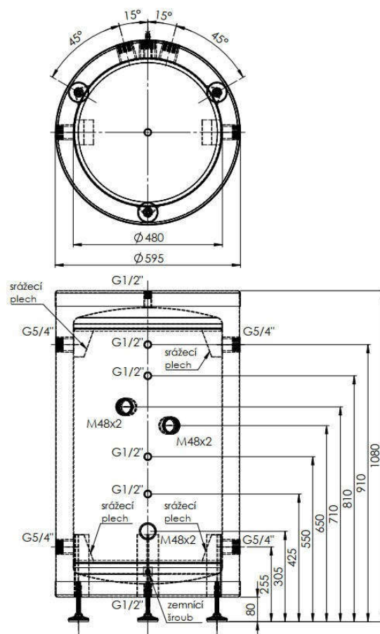
Obr. 4 AKU ST 150 S
