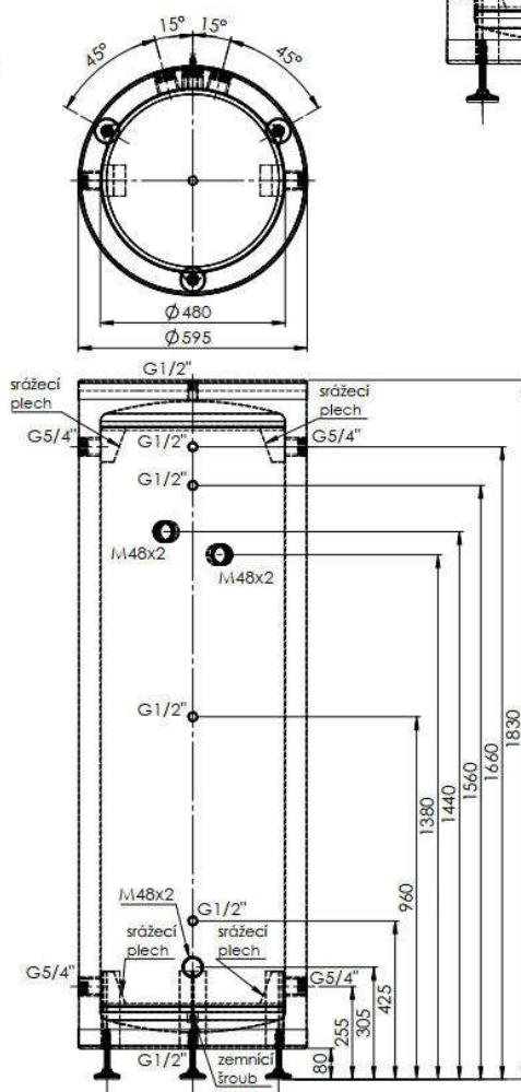
Obr. 5 AKU ST 300 S
